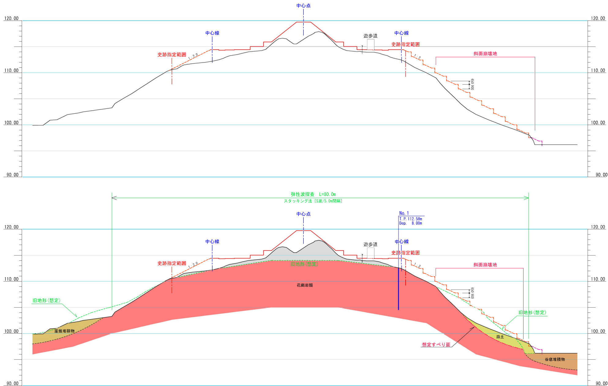
図.2 調査測線簡易横断面図 S=1:300
