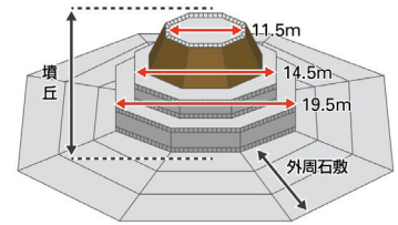
▲墳丘復元図 (関西大学ニュースレター 「Reed」No.64 P.04より転載)
