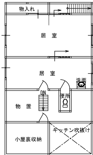
2階 平面図
