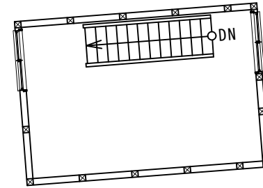
椎茸栽培所 2階 平面図
