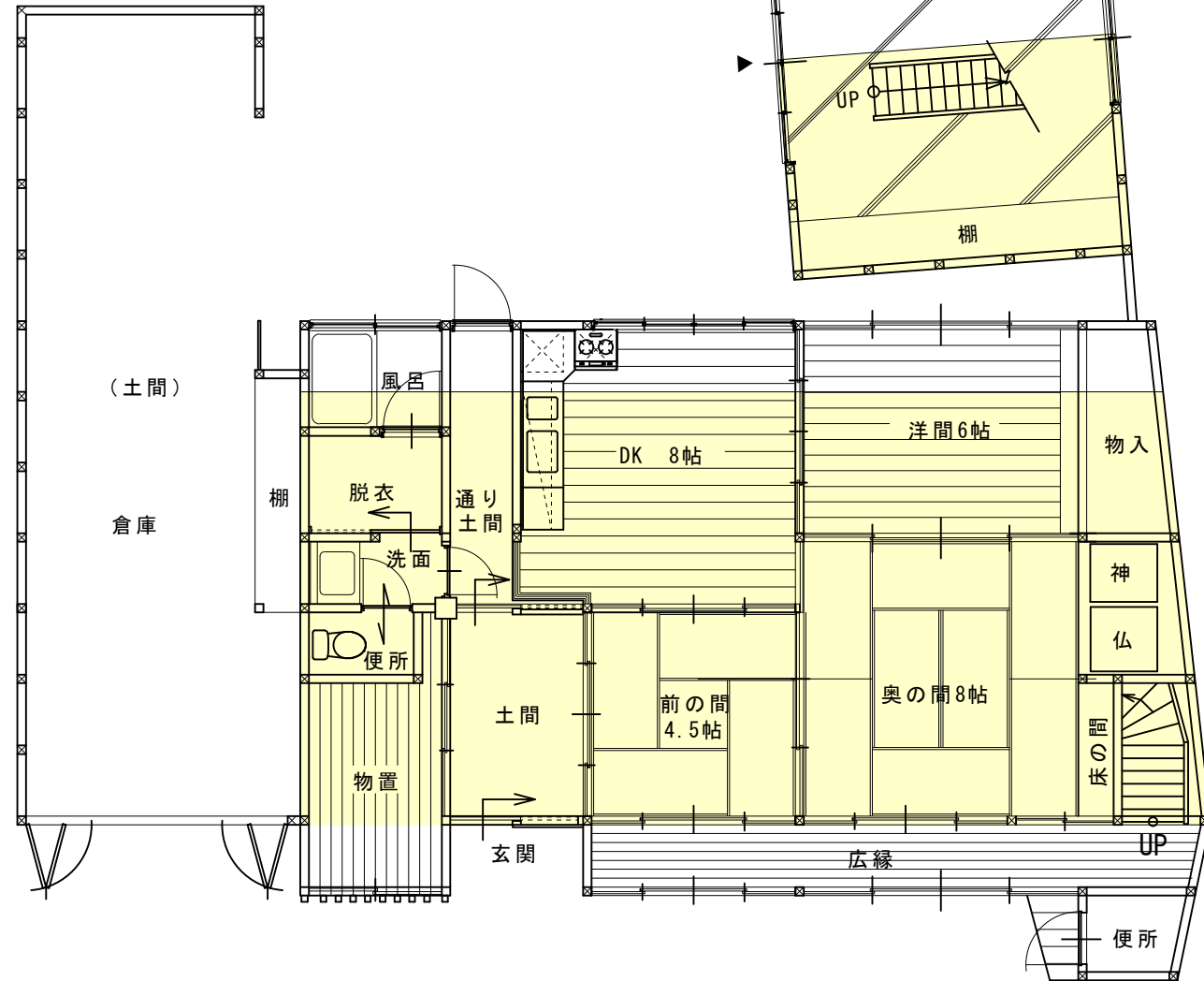
主家 1階 平面図
