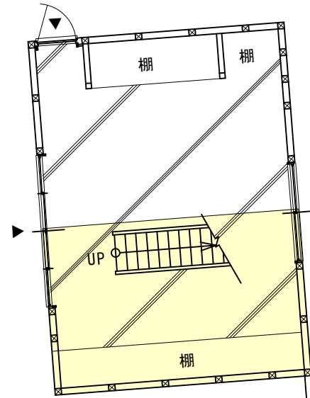
椎茸栽培所 1階 平面図
