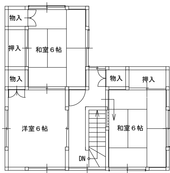
2階平面
