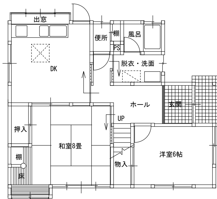
1階平面
